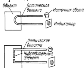
Рис. 1 – Структура волоконно-оптического датчика с изменением характеристик волокну и с изменением параметров передаваемого света
