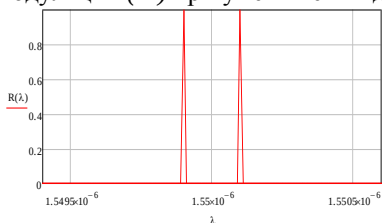
Рис. 3 – Спектр отражения 2\lambda -ВБР
