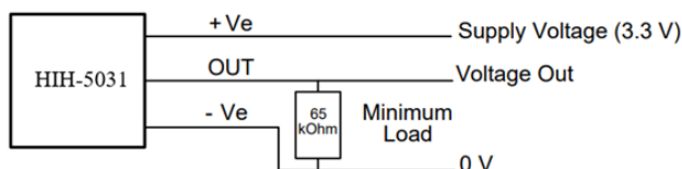
Рис.2 – Типичная схема применения ННН-5031-001
