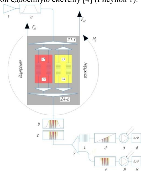
Рис.1 – Оптико-электронная схема системы мониторинга момента рыскания в пятне контакта, где: 1 – широкополосный лазер, 2, 3-4 – АВБС, 5 и 8 – фотоприемники, 6 и 9 – АЦП.
