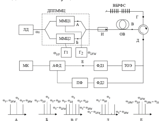
Рис. 1 – Структурная схема ОВА на основе ОДМ с ПН и ВБРФС: ЛД – лазерный диод; И – изолятор; ОВ – оптоволоконно; Г1 – генератор фиксированной частоты; Г2 – генератор сканирующей частоты; ФД1, ФД2 – фотоприемники; ПФ – полосовой фильтр; АФД – амплитудно-фазовый детектор; МК - микроконтроллер
