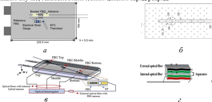
Рис. 1 – Топологии включения ВБР в структуру ЛИБ: точечная наружная (а) и квази-распределенная внутренняя (б); многоточечная наружная (в); многоточечная наружная и внутренняя (г)
