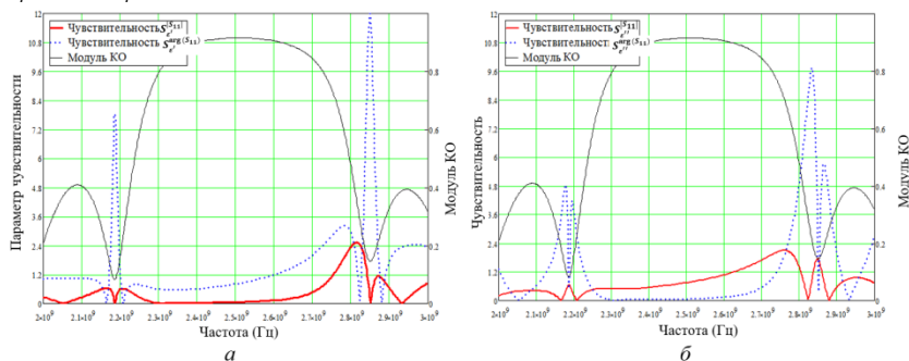
Рис. 3 – Чувствительность модуля и фазы КО при вариации \varepsilon_r' (а) и \varepsilon_r'' (б) в области первой полосы загравждения.
