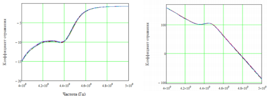
Рис. 2 – Повторяемость эксперимента: модуль коэффициента отражения и фаза коэффициента отражения.
