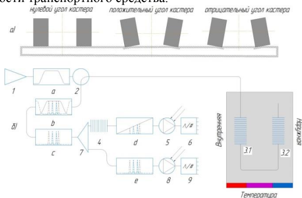
Рис. 1 – а) Схема углов кастера колеса, б) Оптико-электронная система контроля кастера колеса, где: 1 – широкополосный лазер, 2 – циркулятор, 3.1-3.2 – АВБС, 4 – линейный наклонные фильтр, 5 и 8 – фотоприемники, 6 и 9 АЦП, 7 – оптический делитель.
