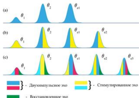
Рисунок 1. Формирование последовательности импульсов фотонного эха при двухимпульсном возбуждении среды. Цветом выделены компоненты, дающие вклад в первого (а), второго (b) и третьего по счёту (с) импульсов эха и имеющие различный физический смысл.
