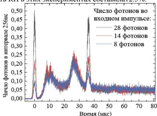
Рис. 2 – Квантовая память в схеме подавленного эха в согласованном оптическом резонаторе в кристалле \text{Tm}^{3+}:\text{Y}_3\text{Al}_5\text{O}_{12} ( c=0.1 ат.%). Черный, синий и красный графики соответствуют разному числу фотонов во входном импульсе. При t=0 приведена непоглощенная часть входного импульса. При t=36 мкс возникают сигналы подавленного эха. Между ними видны сигналы от рефразирующих \pi – импульсов.
